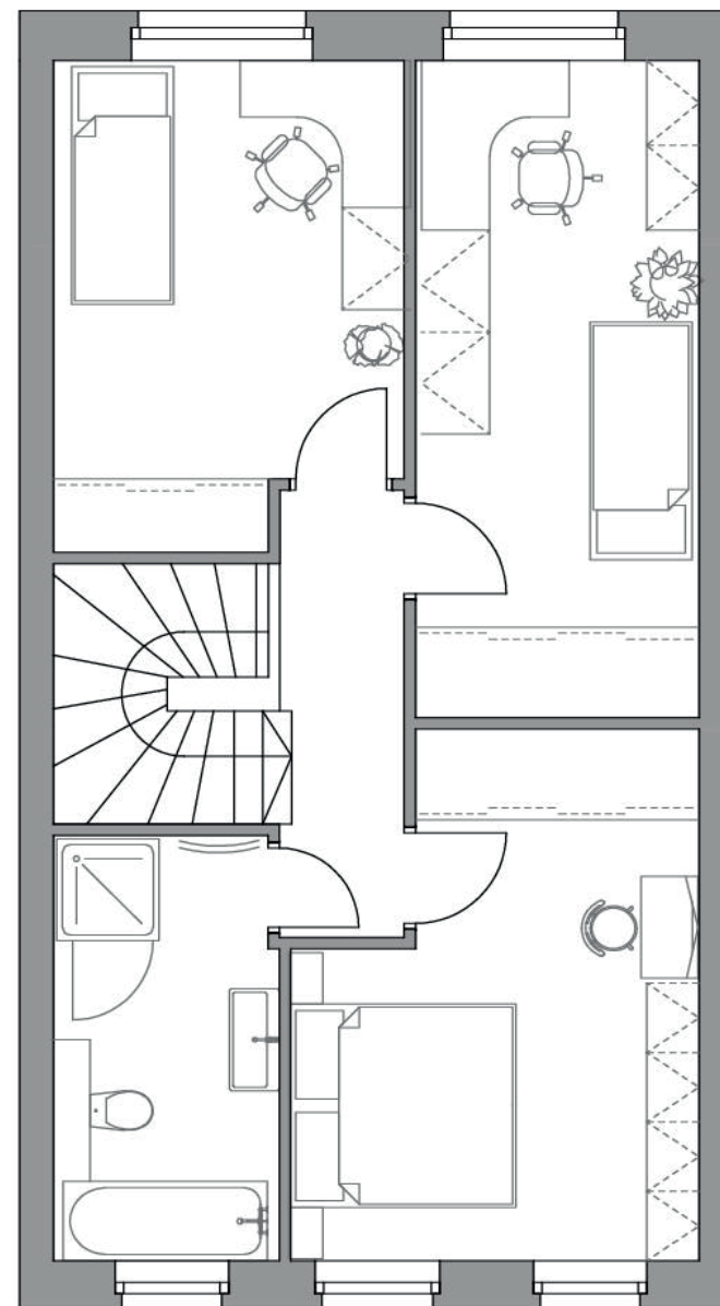
č.19 PŮDORYS PODKROVÍ
