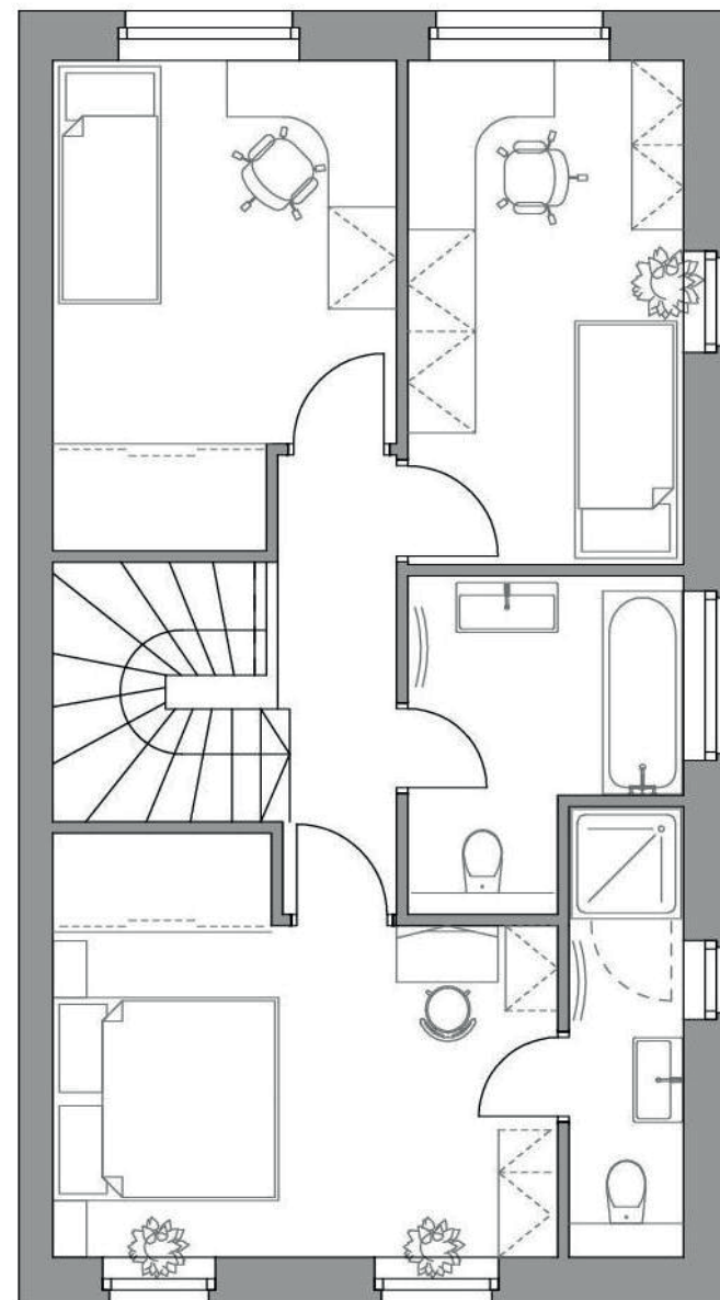
č.18 PŮDORYS PODKROVÍ
